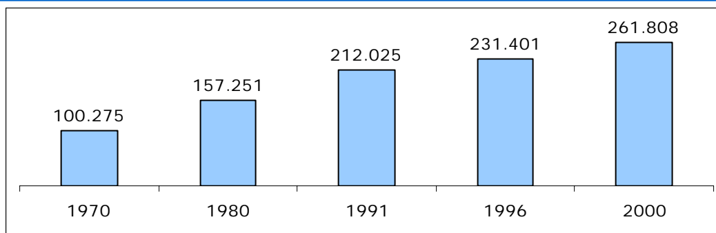
Gráfico 1 - Contagem Populacional
