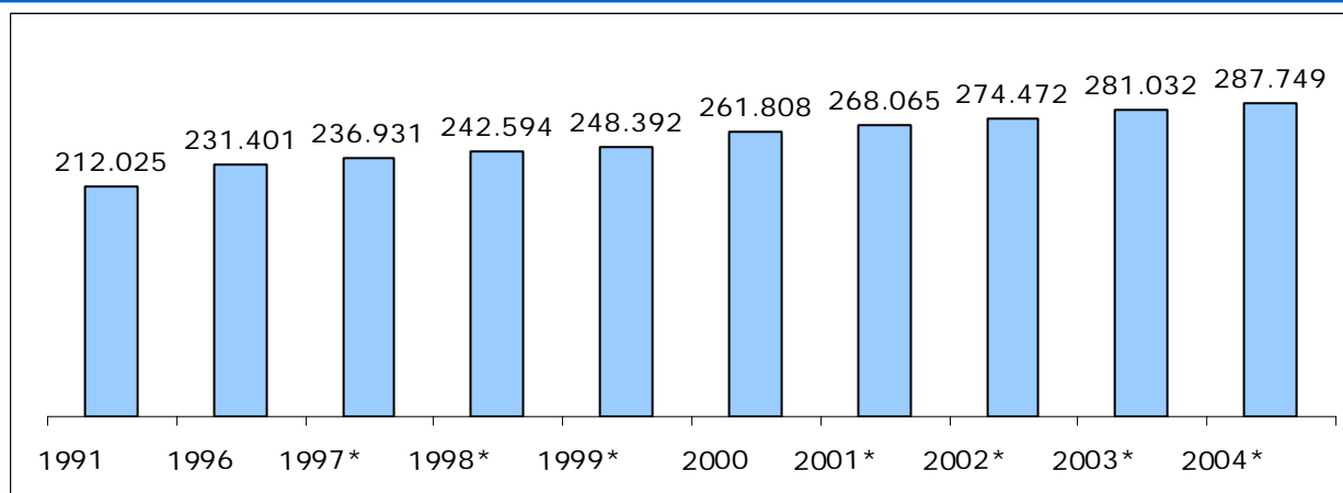
Gráfico 6 – Estimativa Populacional - 2004
